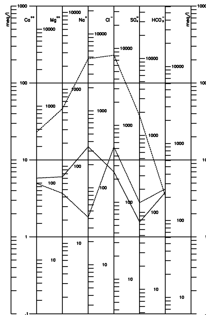
Diagrama de Stiff modificado (Rayado: cambio de escala).
